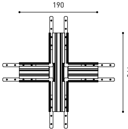
X-JOINT
