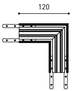
L-JOINT
